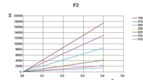
负载/延伸率[%]
