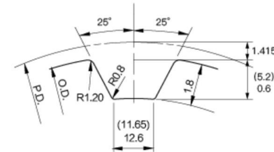
齿形 (ISO标准齿条尺寸)
