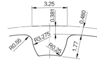
齿形 (ISO标准齿条尺寸)
